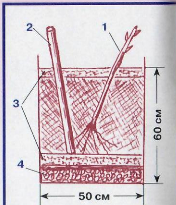
Яма для посадки винограда: 1 - саженец; 2 - труба для полива; 3 - слой песка 10 см; 4 - подушка из битого кирпича
